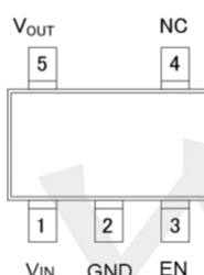
SOT23-5
