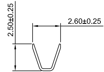
SEC:A-A
