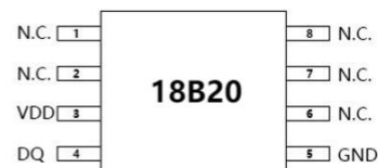
SOP8 (18B20Z)
