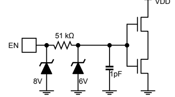
Figure 19d: EN Input
