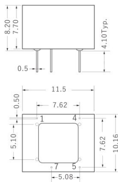
1)外观尺寸(单位:mm,公差:xx±0.25)
