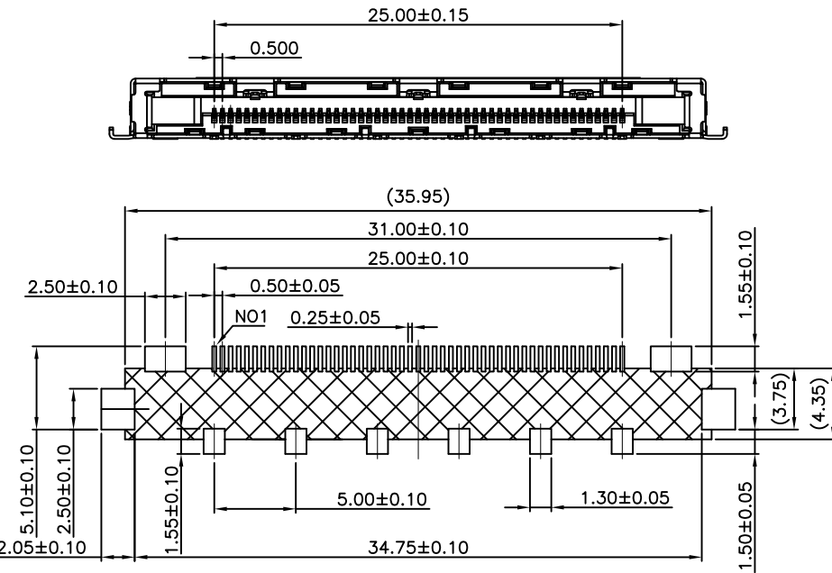
RECOMMEND P.C.B LAYOUT
