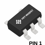
SOT-353/SOT-23-5L
