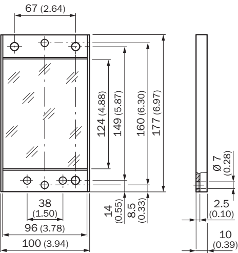
尺寸图 (尺寸单位: mm)
