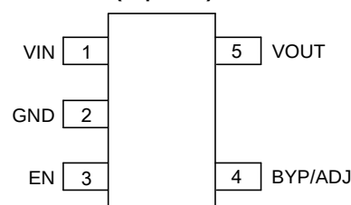
SOT-23-5
