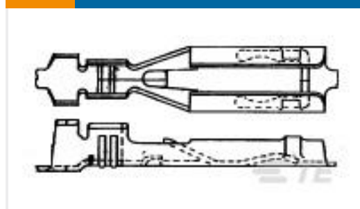
TE Part #66021-3 AMP BLADE RECP MIL PLTD 50 AU
