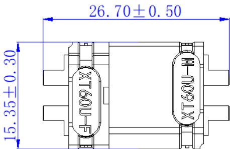
互配尺寸
