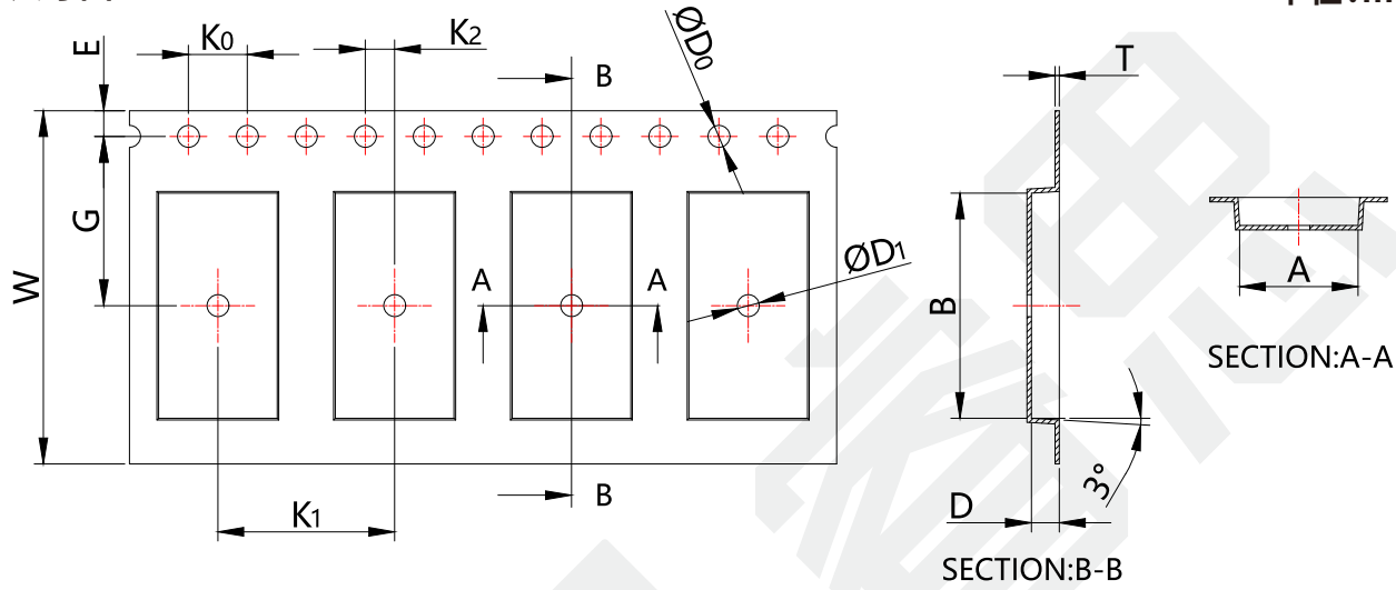
卷编带尺寸图
