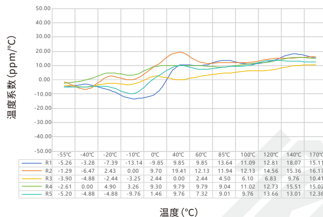
SEWF 系列 5930 规格 1.0mΩ 温度系数实测数据表
