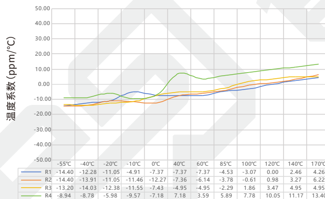
SEWF 系列 5930 规格 2.0mΩ 温度系数实测数据表
