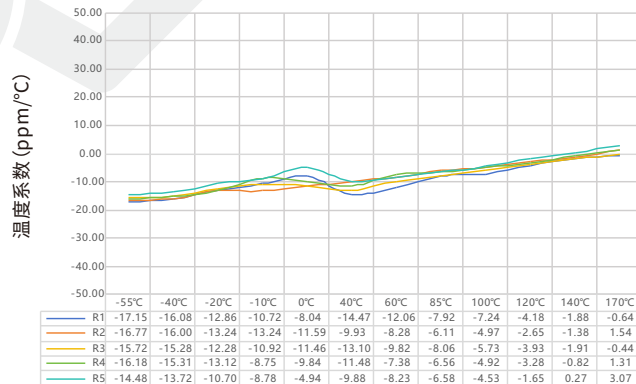
SEWF 系列 5930 规格 3.0mΩ 温度系数实测数据表
