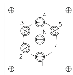
SP5T
