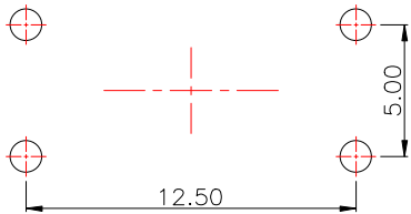
PCB.焊接图
