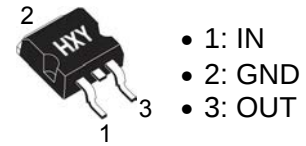
TO-263S (TO-263-2)
