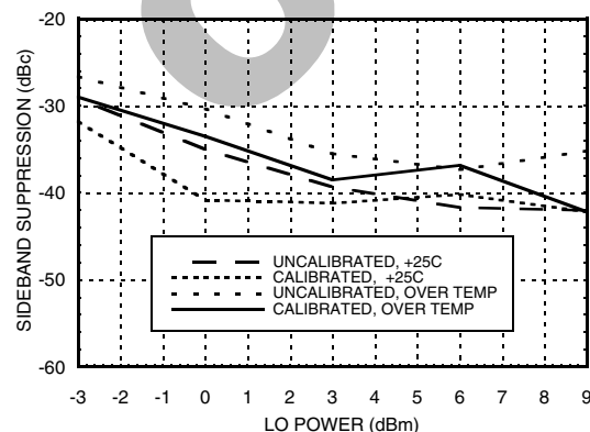
Sideband Suppression* vs. LO Power@ 5800 MHz
