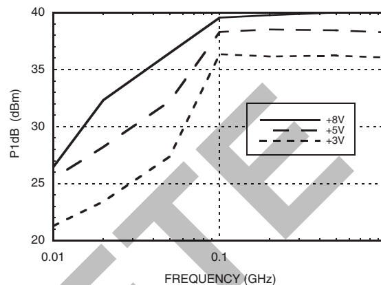
Input P1dB vs. Vdd
