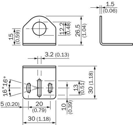
尺寸图 (尺寸单位: mm)
