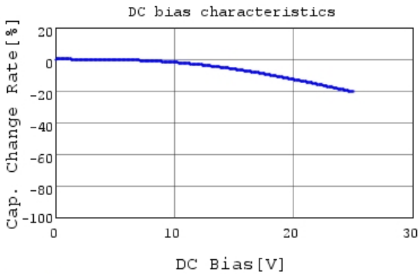
GCJ31CL81E824KA01 C-DC bias capchange, 25.0c
