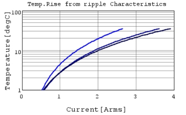
GCJ31CL81E824KA01 Temp.rise — 200kHz —
