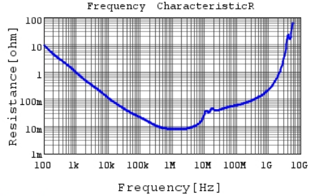
GCJ31CL81E824KA01 R DCOV, 25degC
