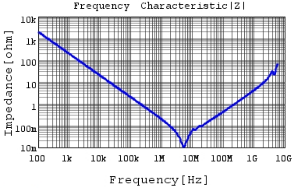
GCJ31CL81E824KA01 |Z| DCOV, 25degC
