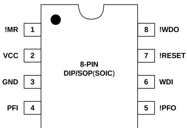
图 3 706R/S/T/J、705/706 的管脚分布示意图
