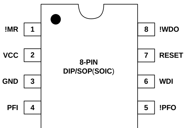
图 2 706P、813L 的管脚分布示意图
