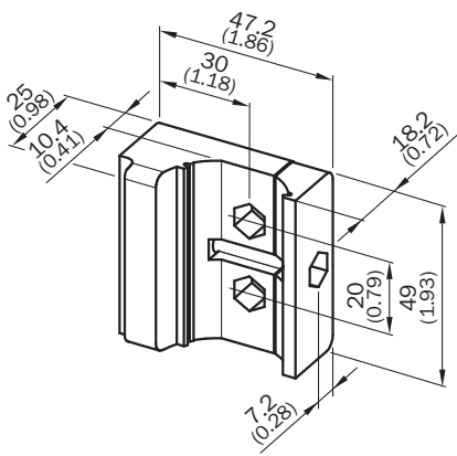
尺寸图 (尺寸单位: mm)
