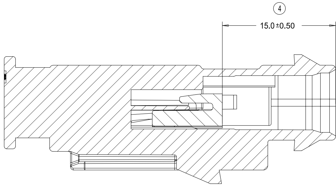
SECTION V-V
