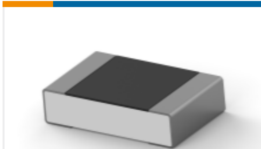
TE Part #1-2176374-0 RQ 0805 133R 0.1% 10PPM 1K RL
