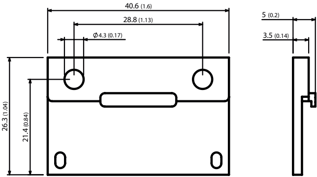
尺寸图 (尺寸单位: mm)
