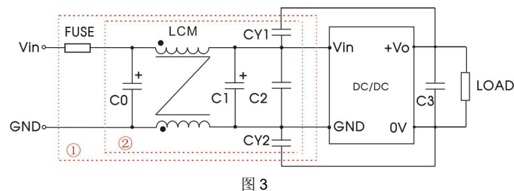
图3中第①部分用于EMC测试;第②部分用于EMI滤波,可依据需求选择。
