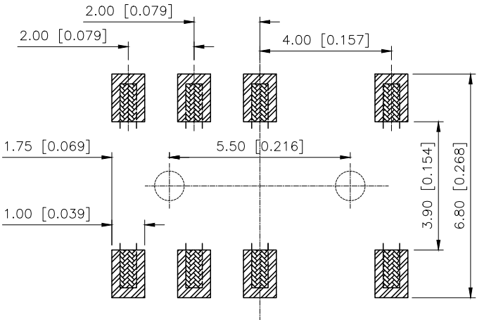
安装图 (PCB LAYOUT PLAN)
