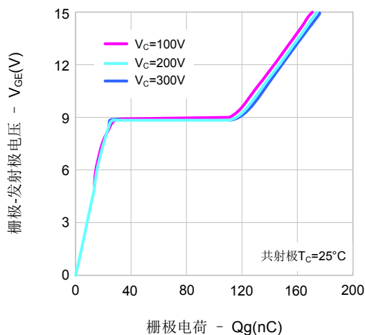
图8. 栅极电荷
