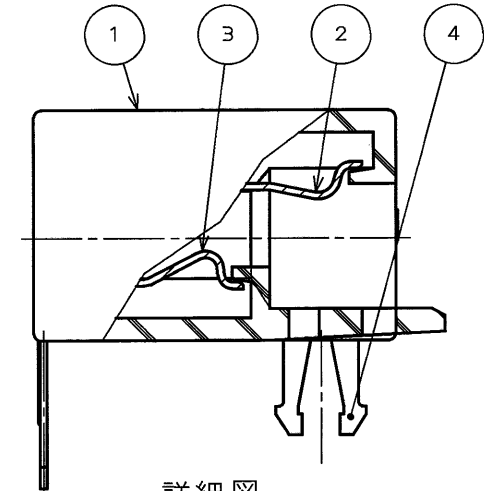
詳細図 (尺度 5/1)
