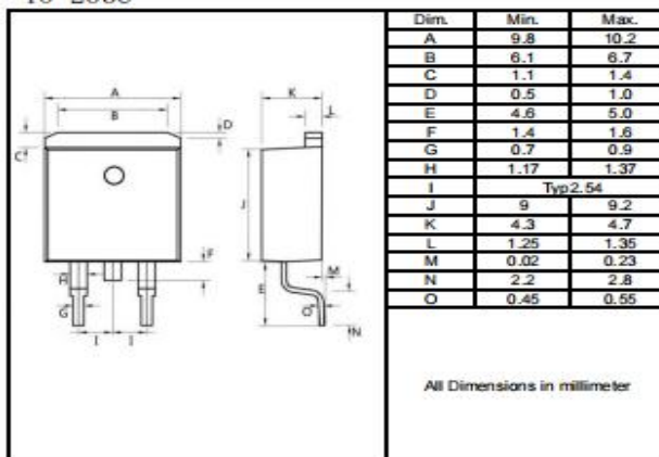
TO-263C
