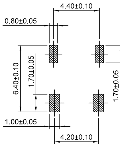
P.C.B LAYOUT
