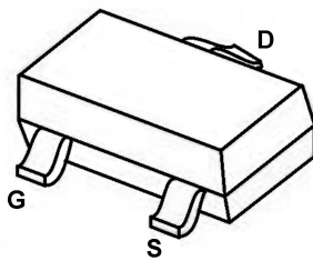
SOT-23-3L
