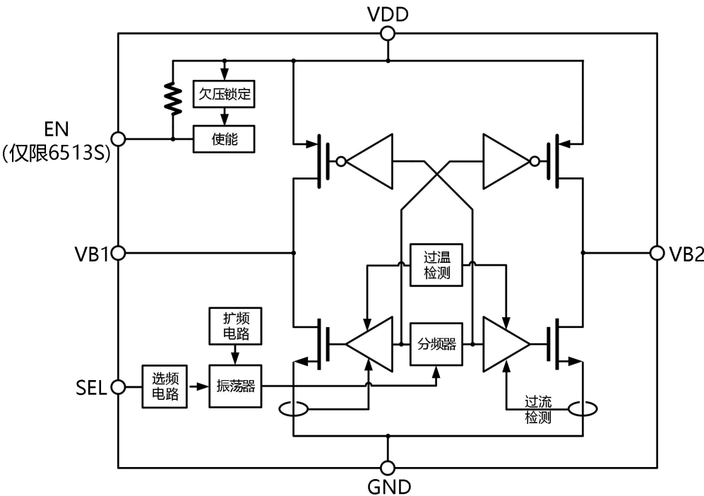
图 7.1 原理示意图
