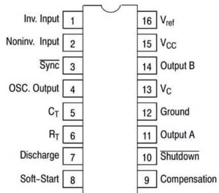
引脚图
