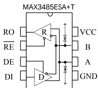
图 1 MAX3485ESA+T 引脚分布图
