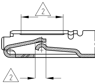
断面 C-C SECT C-C
