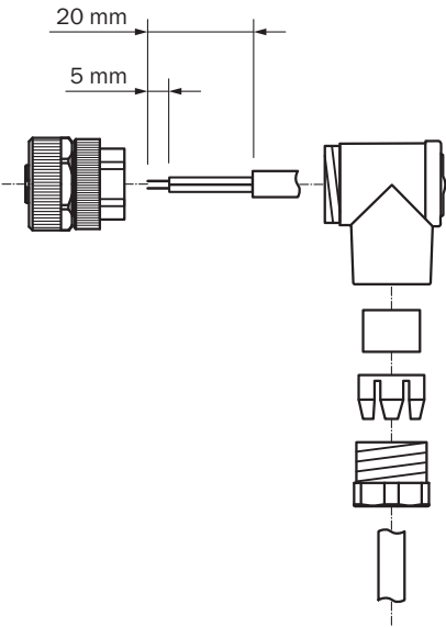
安装图纸
