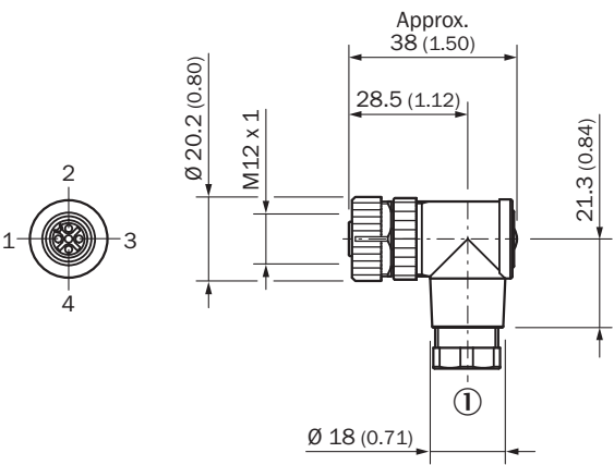
尺寸图 (尺寸单位: mm)
