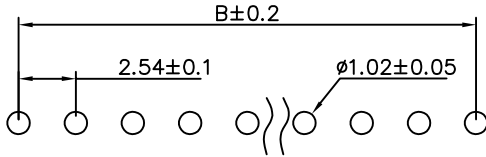
P.C.B LAYOUT
