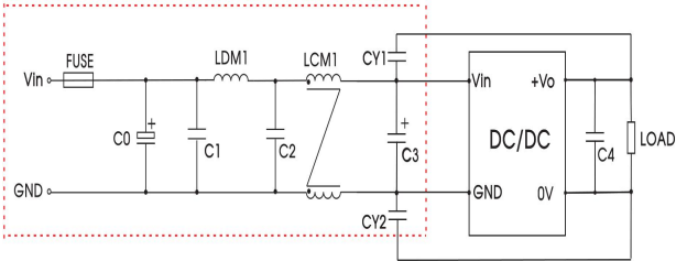
图 3 注：图 3 中红框部分用于 EMS 测试和 EMI 滤波。
