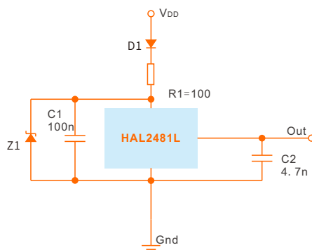
反向保护应用电路
