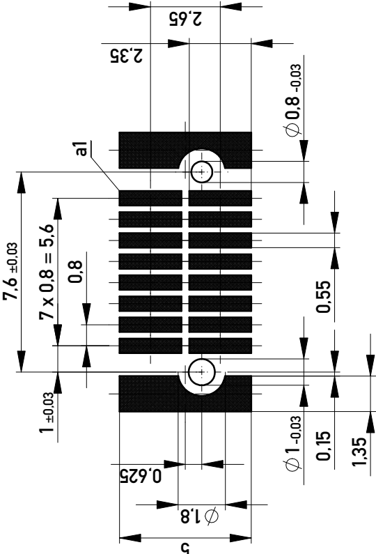
Leiterplatten-Layout Vorschlag für SMT PCB-Layout Proposal for SMT
