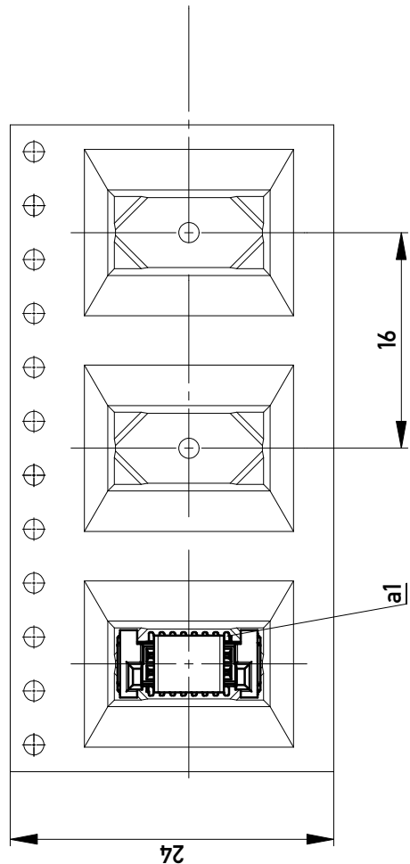
Abspulrichtung - Reel off Direction
