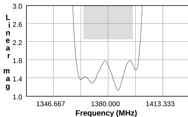
S11 VSWR
