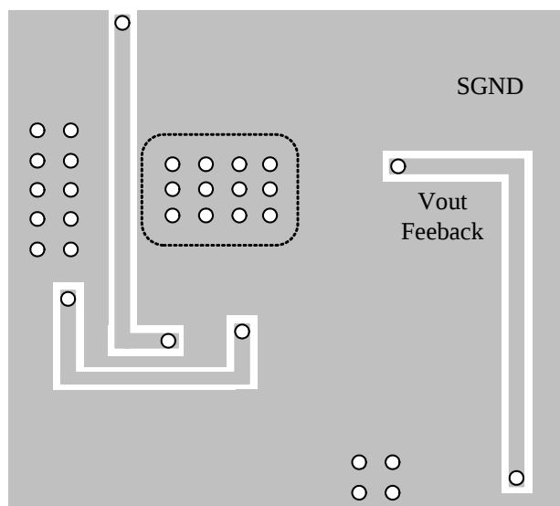
Bottom Layer
