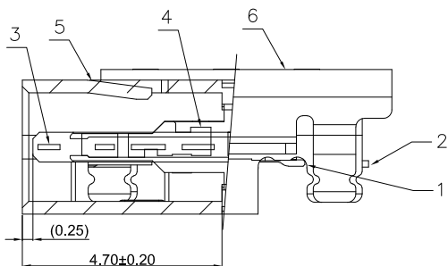
SECTION A-A(剖视图A-A) SCALE 2:1 (比例 2:1)
