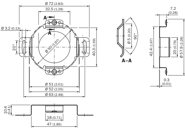
尺寸图 (尺寸单位: mm)
