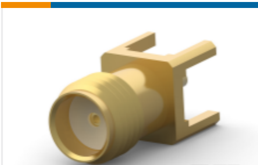
TE Part #5-1814832-2 SMA Str PCB Skt GZD
