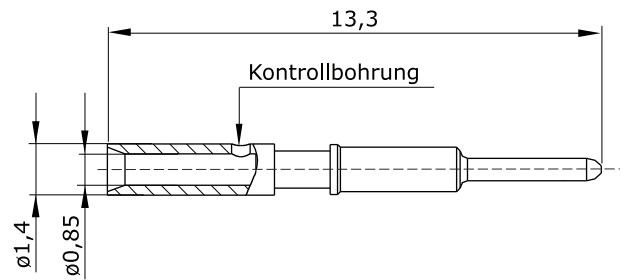
Hauptabmessungen Kontaktstift
