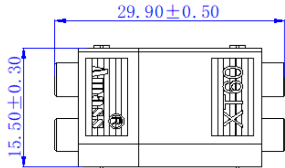
互配尺寸
