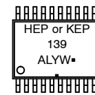
TSSOP-20 WB
