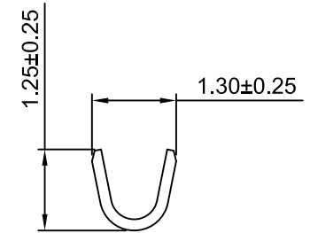
SEC:B-B
