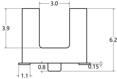
正面图
