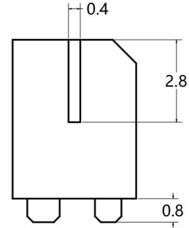
侧面图
