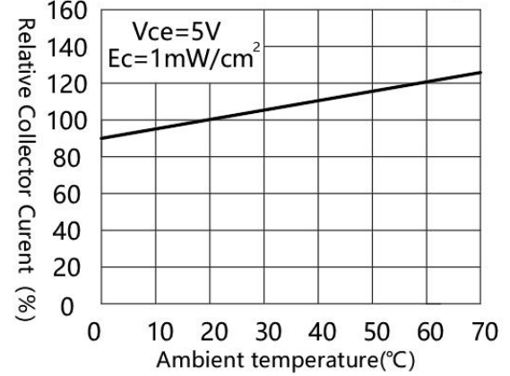
相对集电极电流与环境温度的关系
